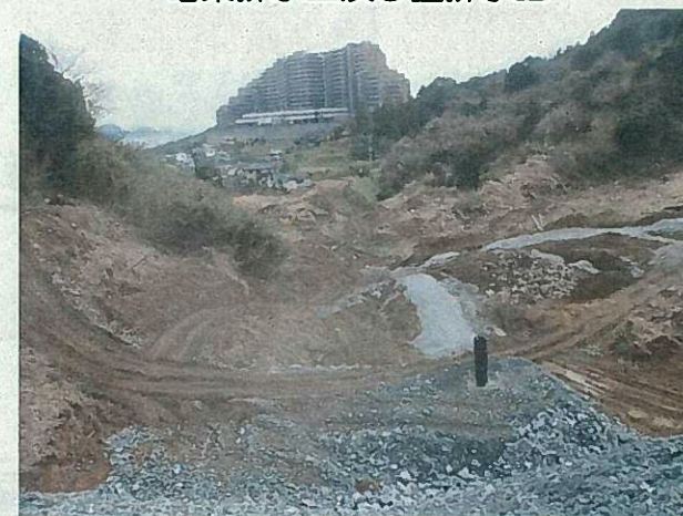
暗渠排水工及び縦排水工
